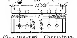
Figs. 1991-1992. Carry-iron.
